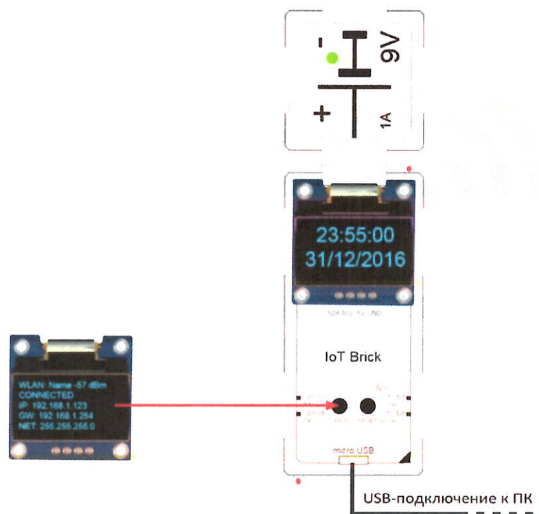
Рисунок 3.9.2 – Схема подключения
