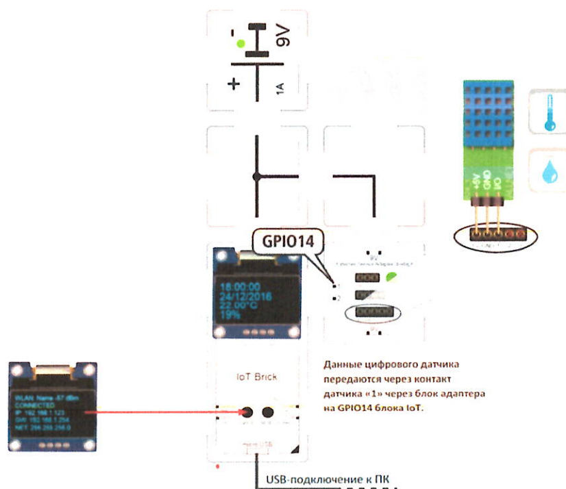
Рисунок 2.1 – Схема измерения температуры и влажности
