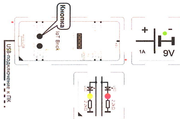
Рисунок 3.8.2 – Схема подключения
