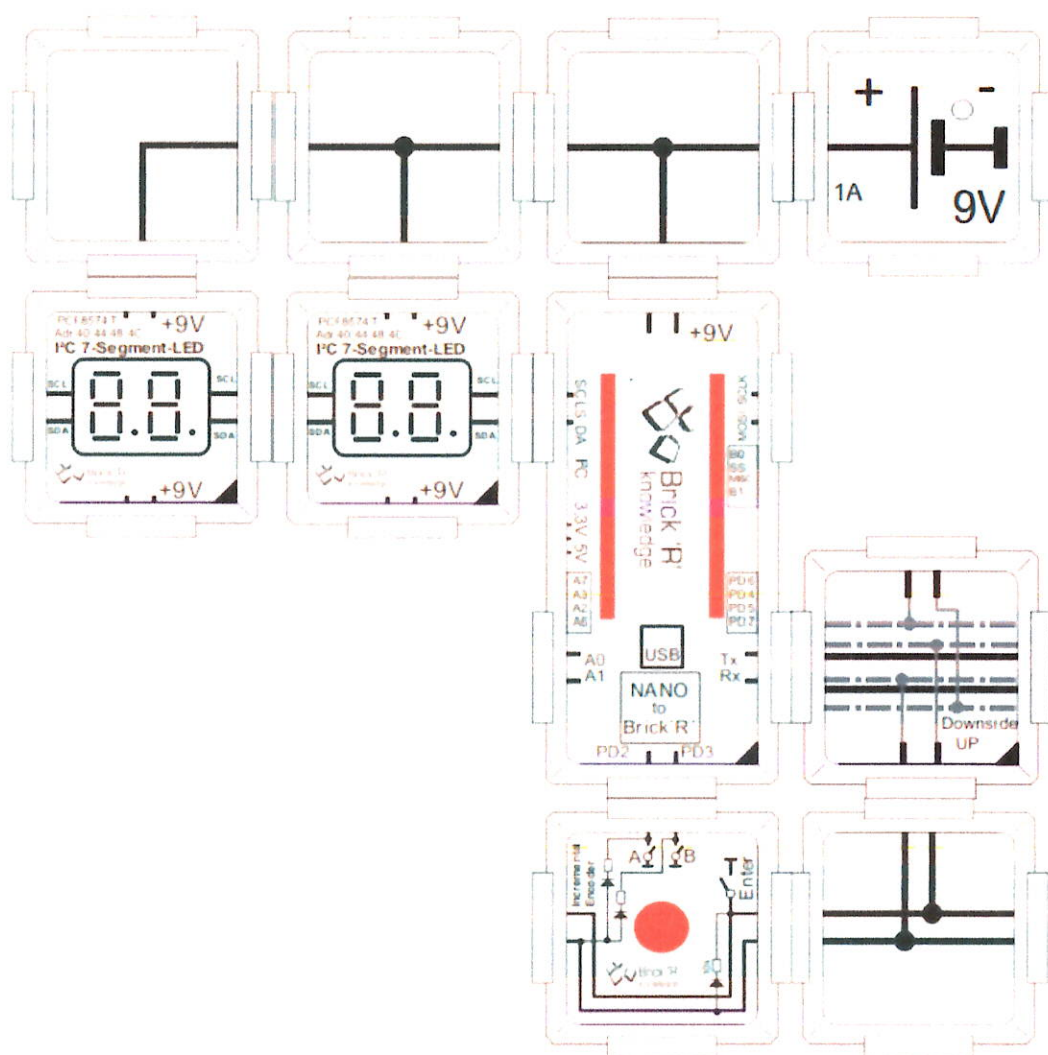
Рисунок 3.5.1 – Схема подключения
