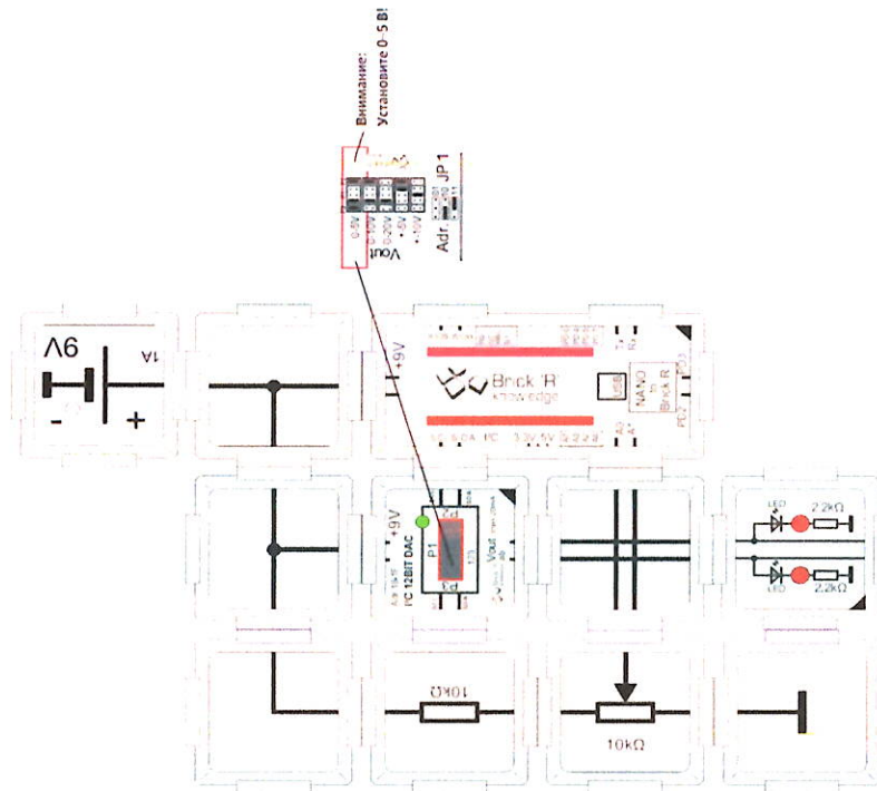
Рисунок 3.7.1 – Схема подключения
