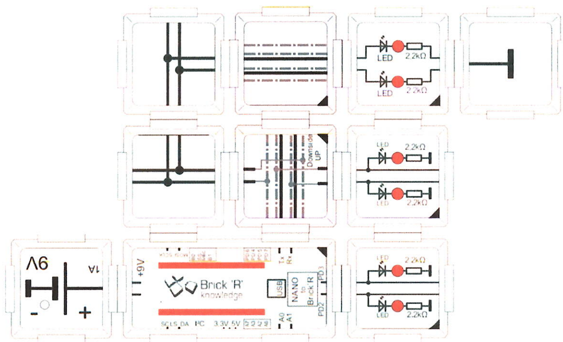
Рисунок 3.1.1 – Схема подключения
