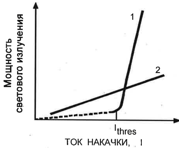
Рисунок 1. Ватт-АХ лазерного диода (1) и светодиода (2).
